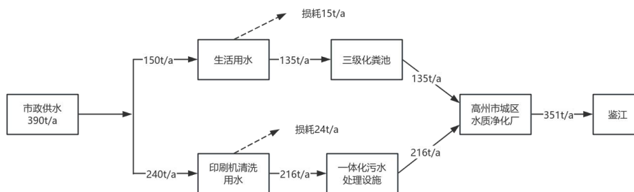
图 2-1 水平衡图单位：t/a
