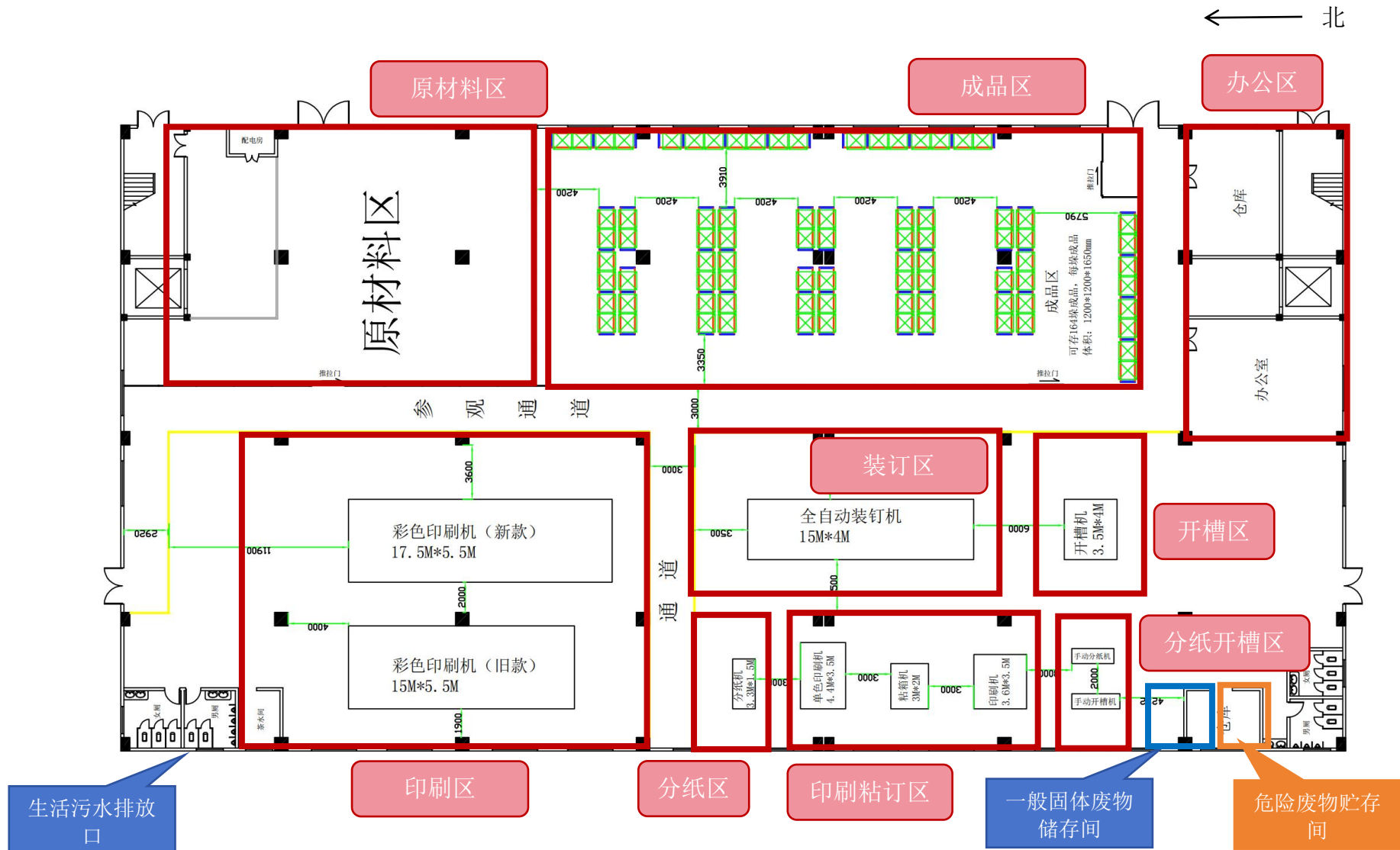
附图 3 一层厂房平面布置图
