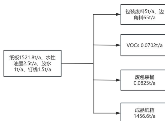
图 2-1 物料消耗平衡图
